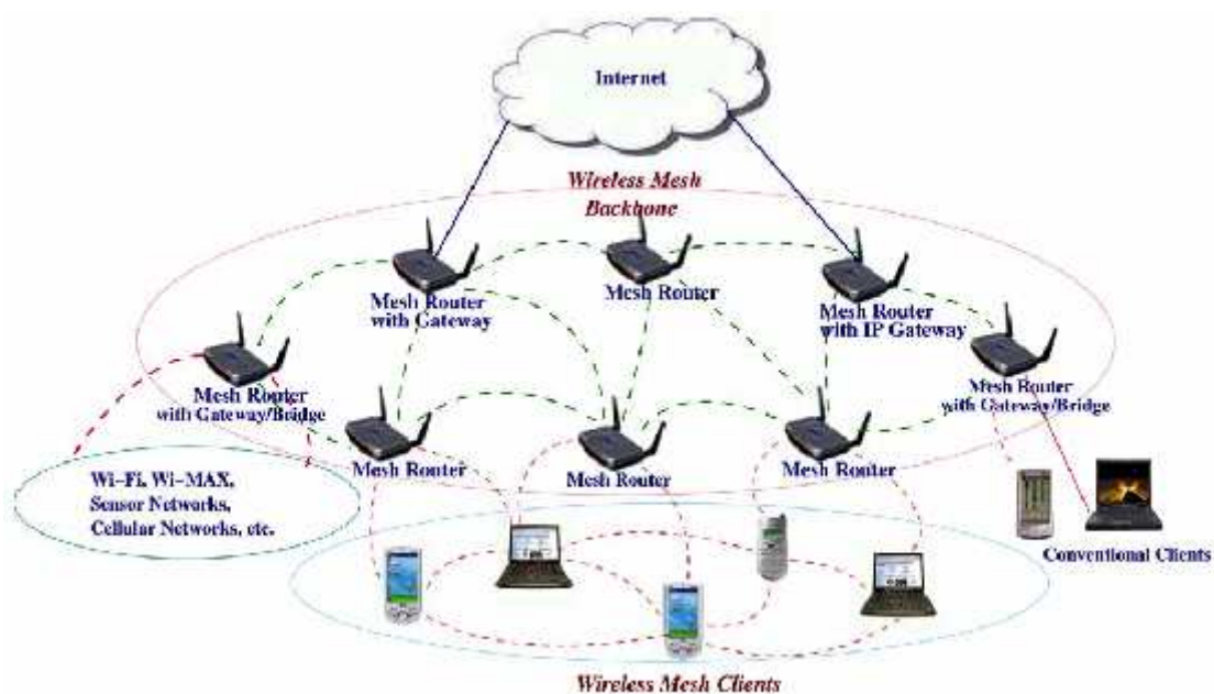
Figura 28 – Rede Mesh com múltiplas tecnologias [Akyildiz et al. 2005]
